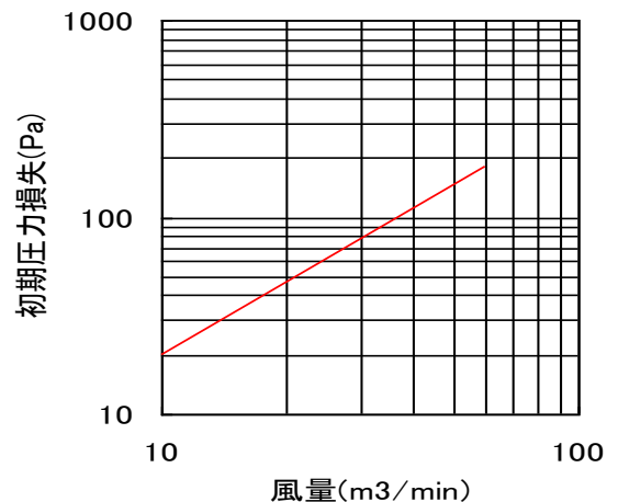
フィルタ厚み 290mm
