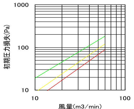
フィルタ厚み 65mm
