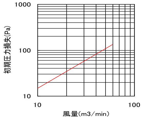
捕集効率 90%
